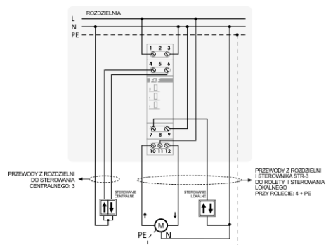
Przykład okablowania: tryb z jednym przyciskiem lokalnym
