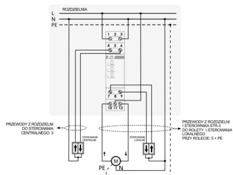
Przykład okablowania: tryb z dwoma przyciskami lokalnymi
