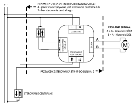
Przykład okablowania: tryb z dwoma przyciskami lokalnymi
