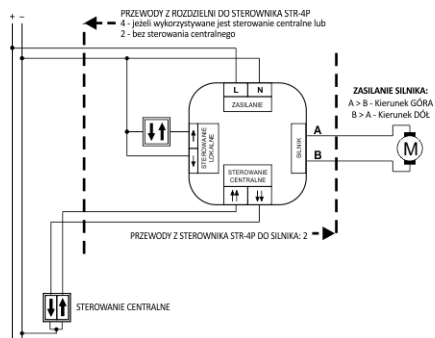
Przykład okablowania: tryb z jednym przyciskiem lokalnym
